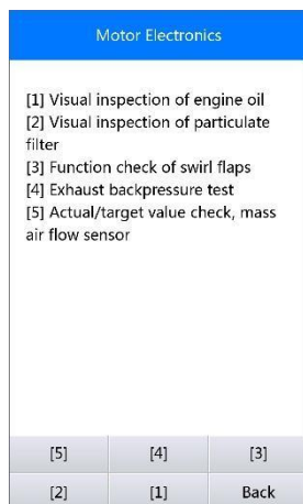
La Figure 5-32 tests du filtre à particules
